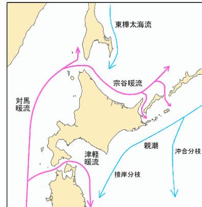
図 13-2 対馬海流の流路
