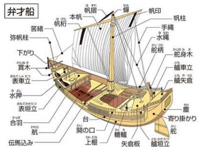
図 4-2 弁才船の部材名称（出典：goo 辞書）
