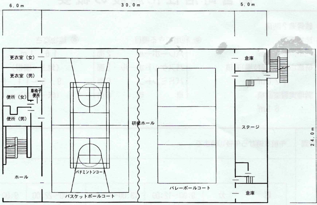
2階平面図
