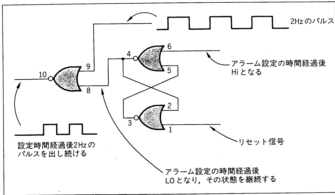
《第5図》MC14001Bの動作説明
