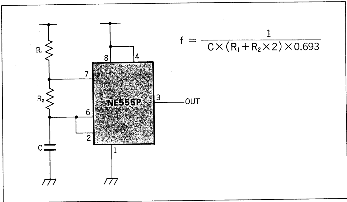
《第4図》NE555Pの発振周波数
