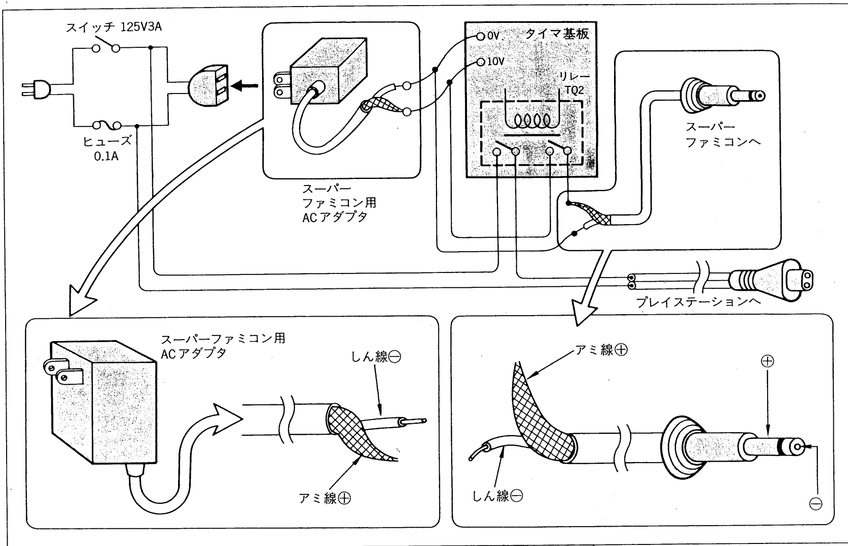
《第2図》ゲーム機の電源はこのようにしたほうが安全
