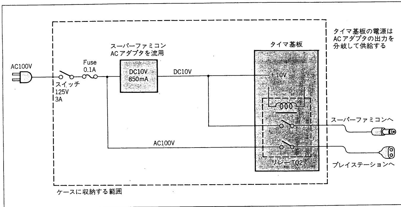
《第1図》全体の接続図
