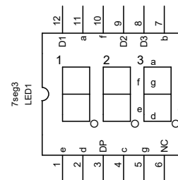
カソードコモン7セグLED C-533R
