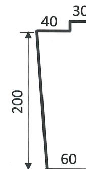
断面図 B-B
