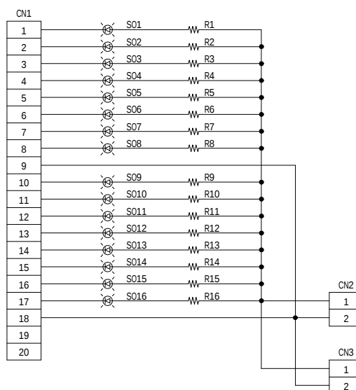
LED基板回路
