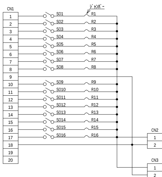
SW基板回路
