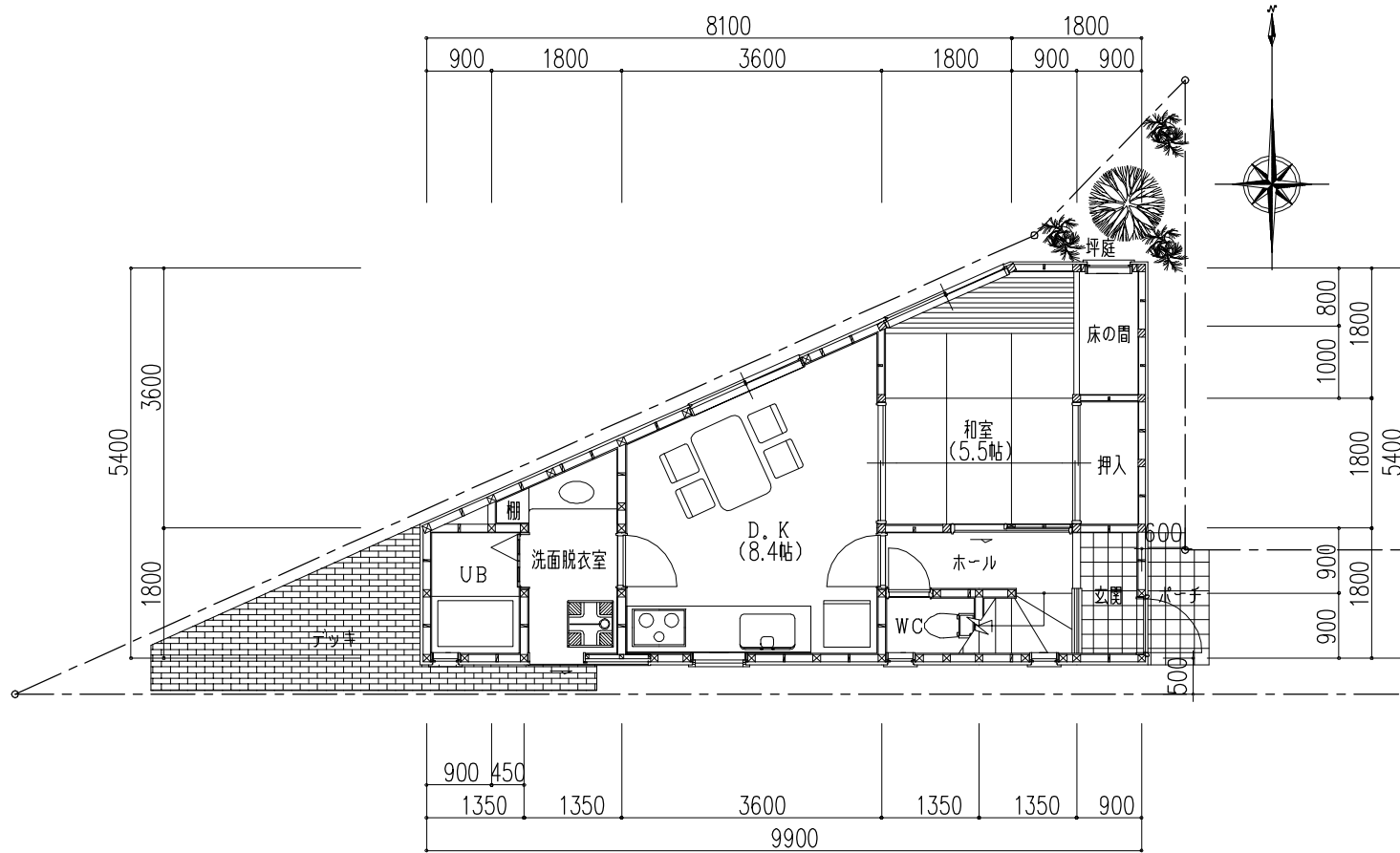
1階平面図 1:100
