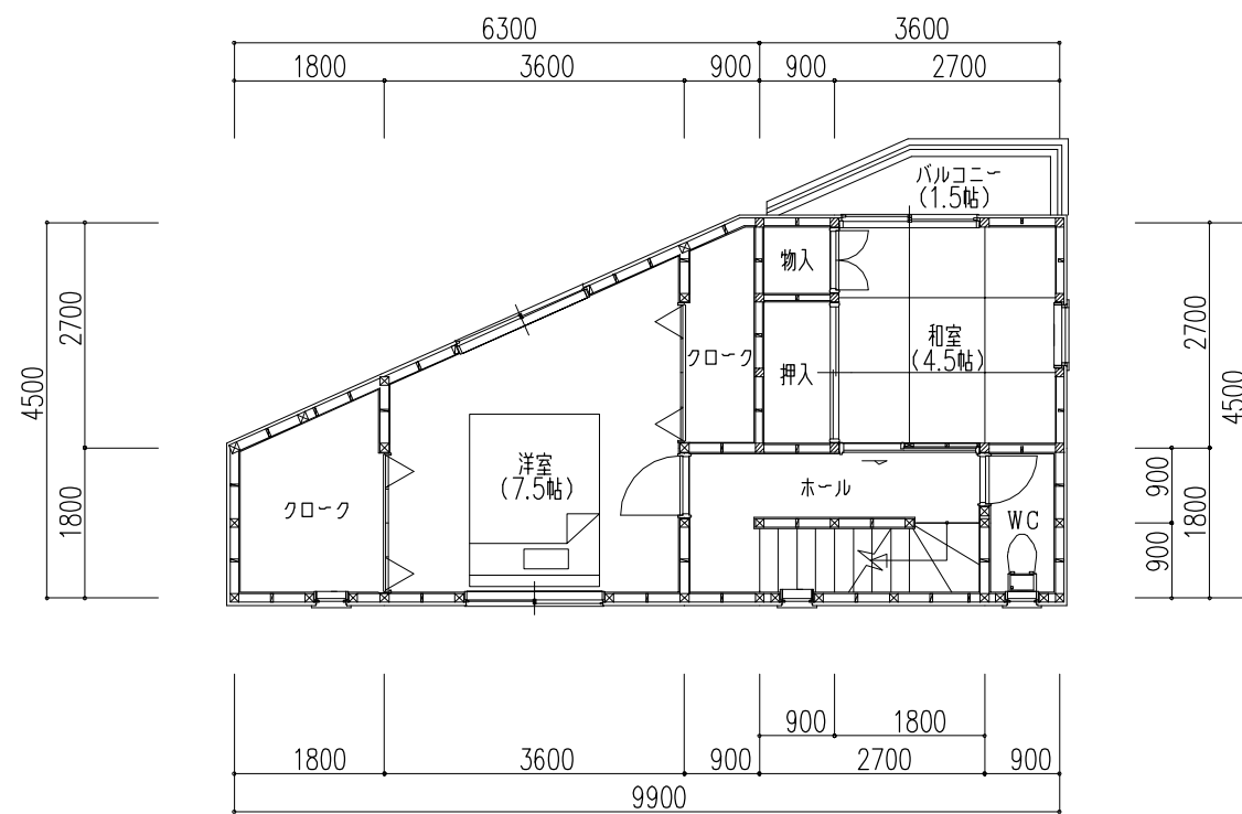
2階平面図 1:100
