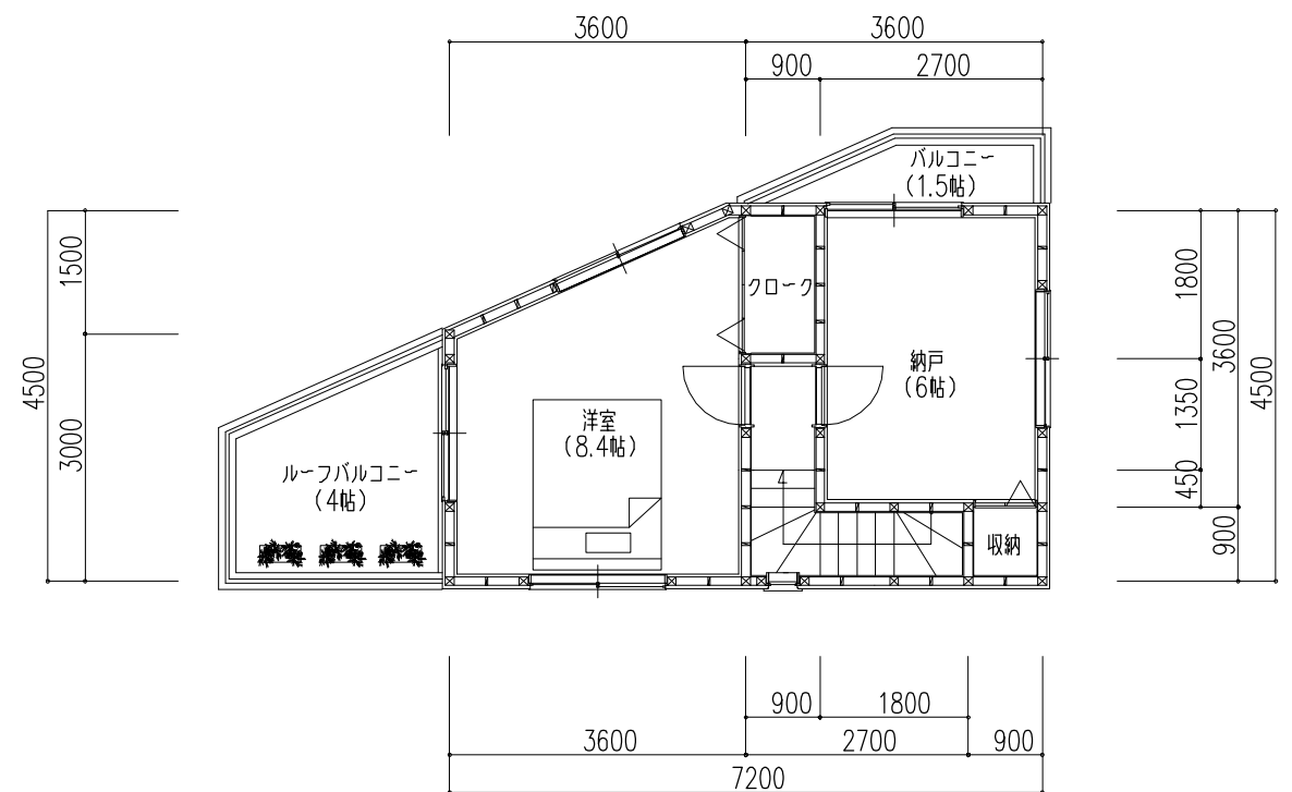
3階平面図 1:100
